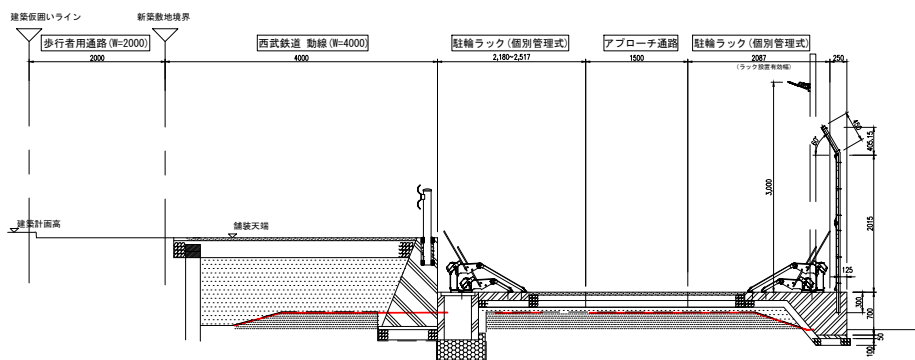
標準断面図
