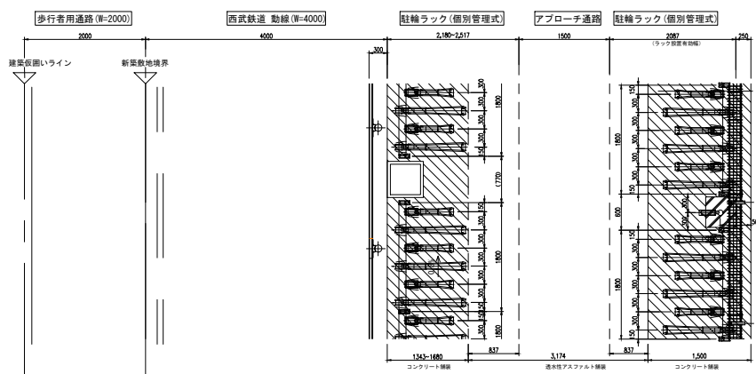
標準平面図
